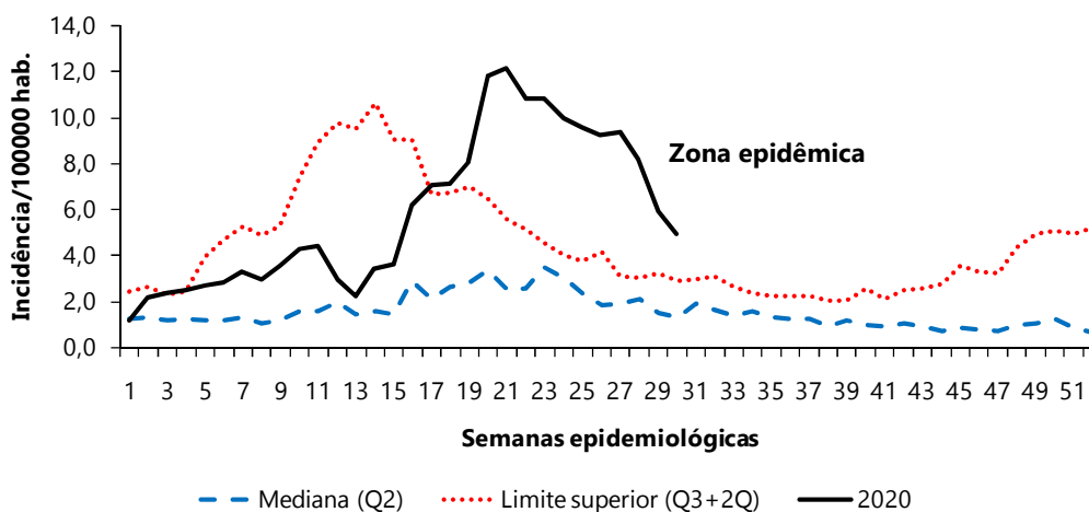
Figura 7 - Diagrama de controle (distribuição interquartil) dos casos prováveis de dengue. Pernambuco, SE 30/2020
