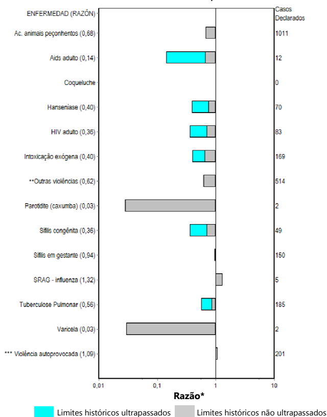
Figura 2 - Comparação dos casos de DNC confirmados e priorizados na quadrissemana (SE 27 a 30) com seu comportamento histórico. Pernambuco, 2020
