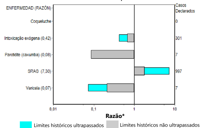
Figura 1 - Comparação dos casos de DNC notificados priorizados na quadrissemana (27 a 30) com o seu comportamento histórico. Pernambuco, 2020
