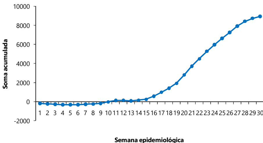
Figura 5 - Carta controle de somas acumuladas dos casos prováveis de dengue. Pernambuco, SE 30/2020
