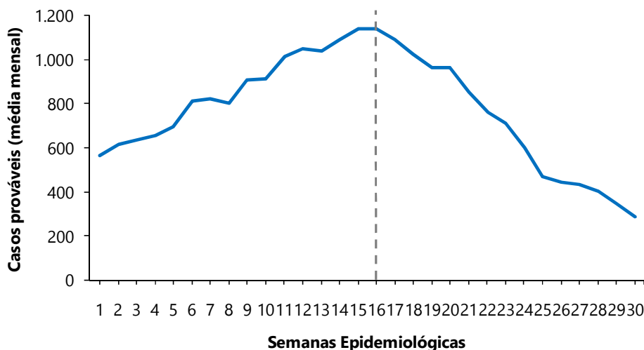
Figura 4 – Registro médio semanal de casos prováveis de dengue. Pernambuco, 2011-2020 (SE 30)
